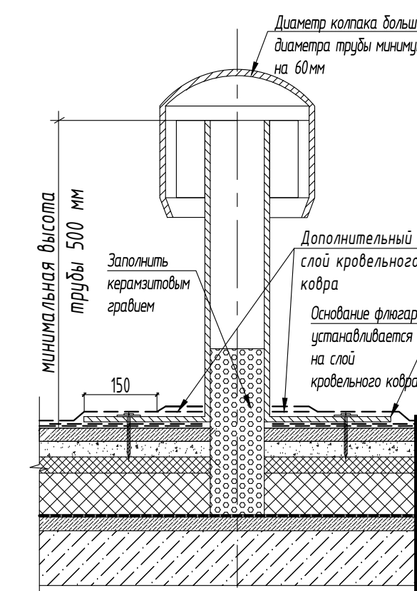
Устройство кровельного азуратора
