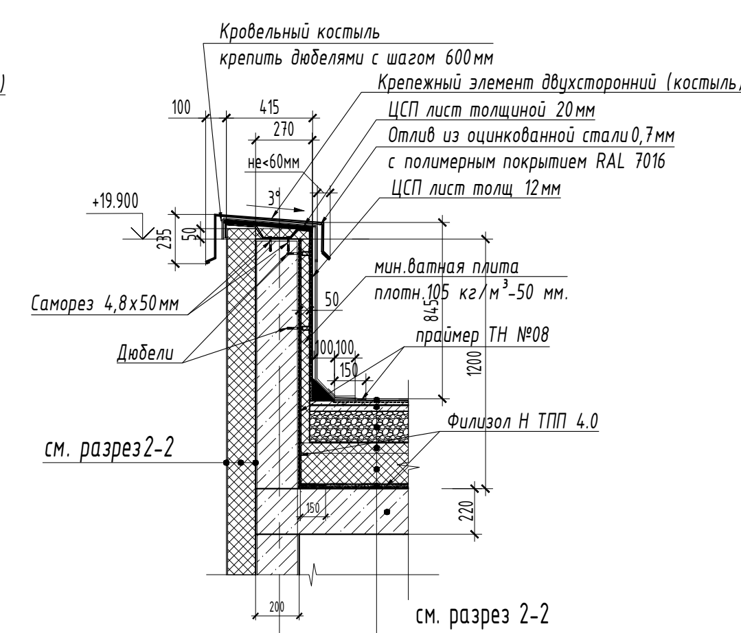
Парапет из желез
