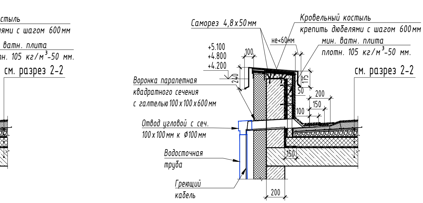
Устройство водоотведения через парапет железобетонный
